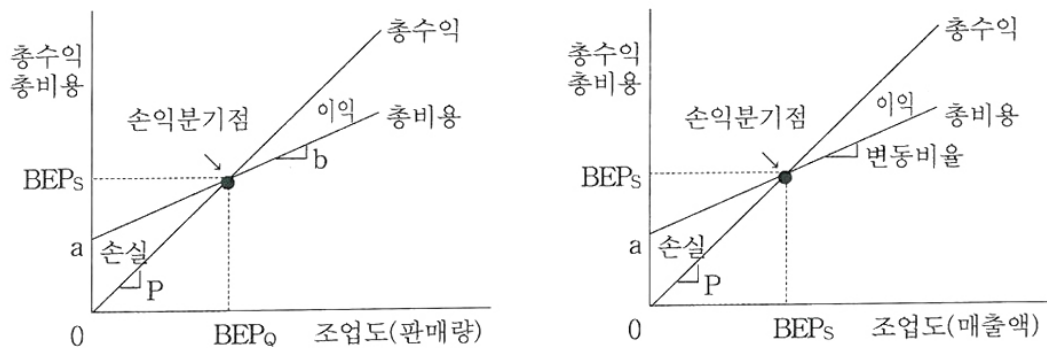
그림 4-1 > CVP도표
